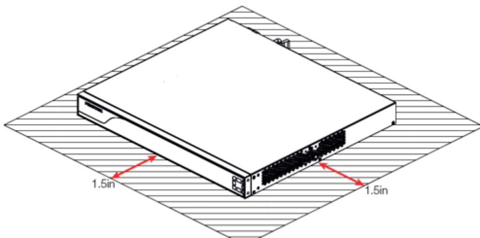
图 2-1 RG-M5100E 通风方式示意图
