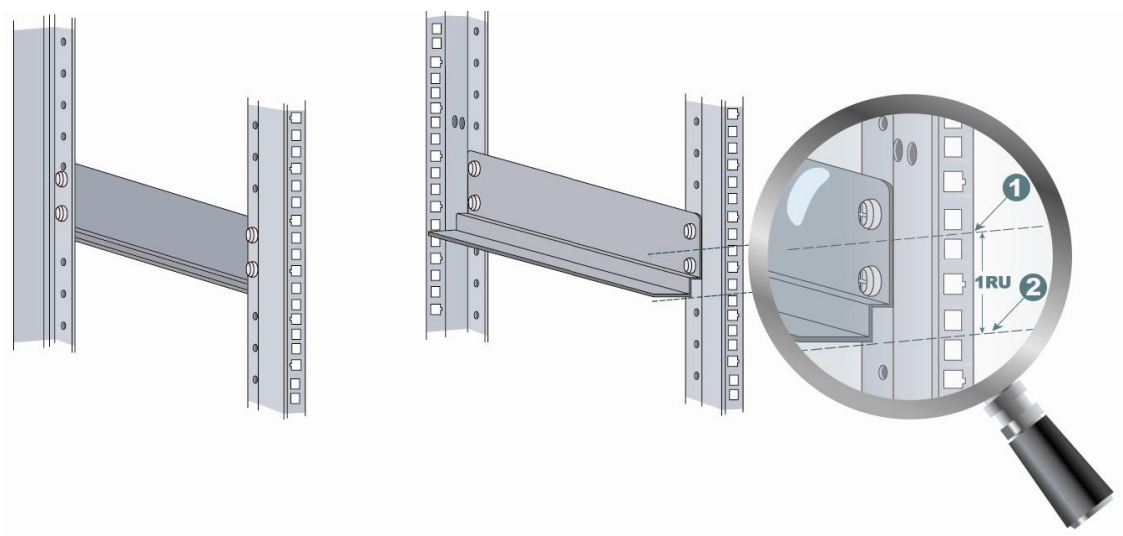
图 3-1 滑道示意图
