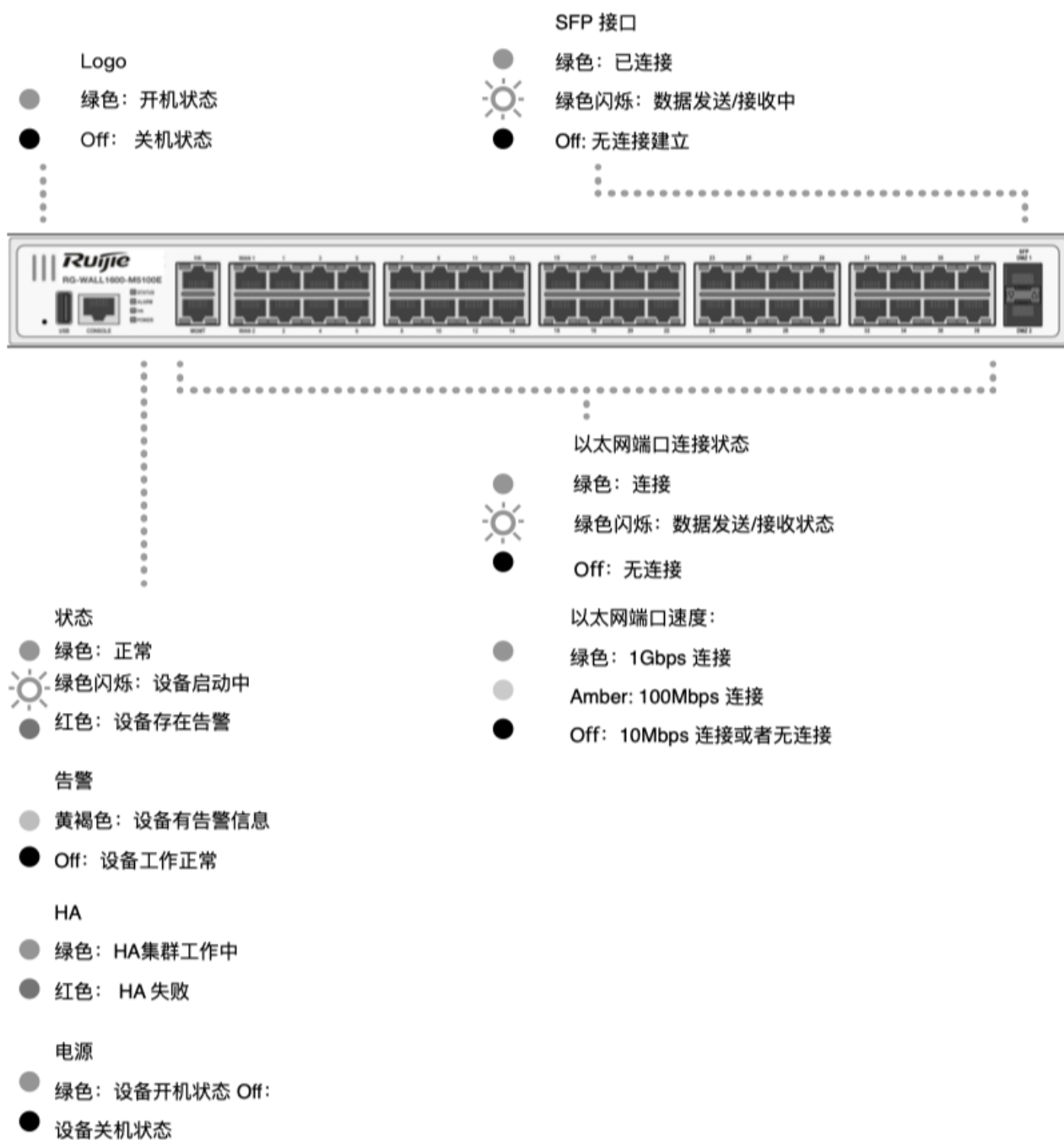
图 5-1 RG-WALL1600-M5100E 的指示灯示意图
